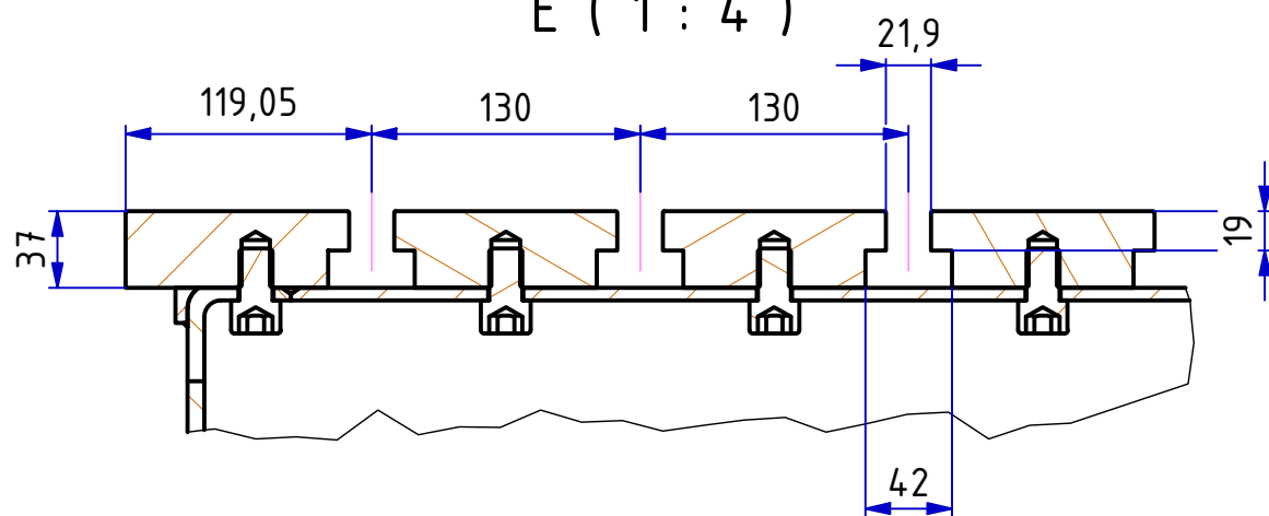
E ( 1 : 4 )
